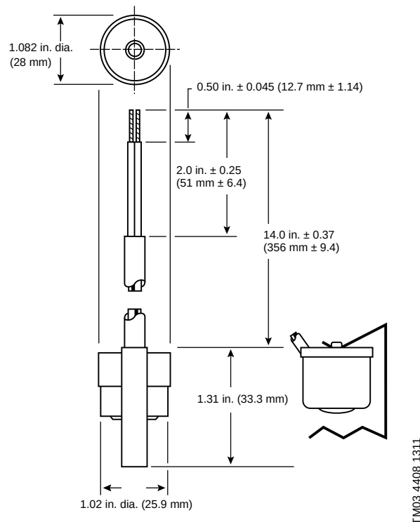
Fig. 14 AquaStat dimensions
